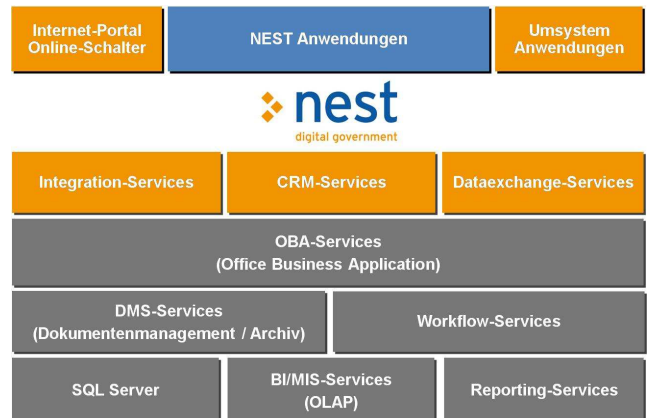
Systemaufbau
